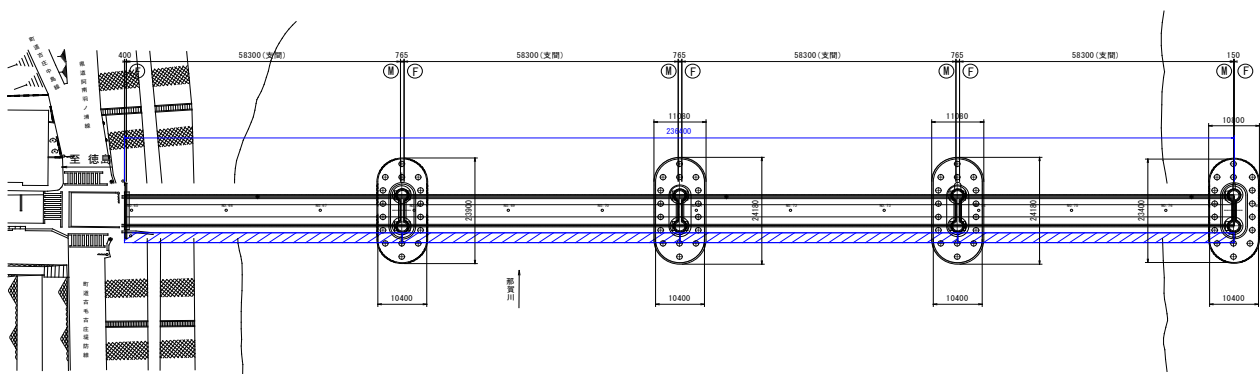
图-2 平面图
